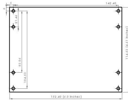
MIT Rocket Team USLI - Avionics Tray 2
