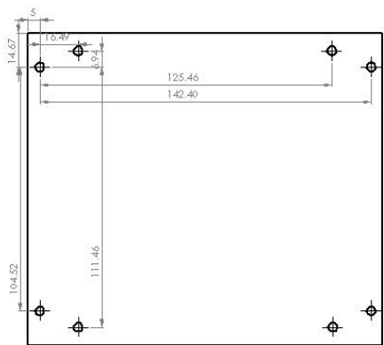
MIT RT USLI A volincs Tray 1
